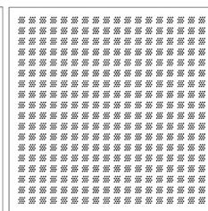
R3 (d=1,5 мм) мини-квадраты (14x14 мм)
